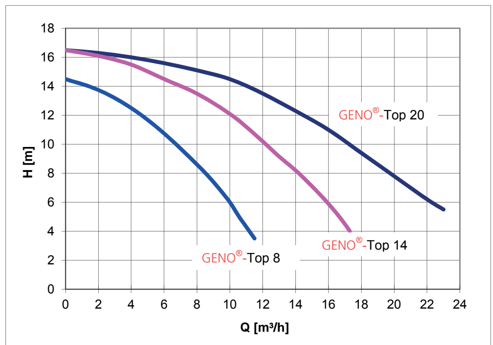
Abb. E-2: Pumpenkennlinien GENO®-Top 8,14 bzw. 20
