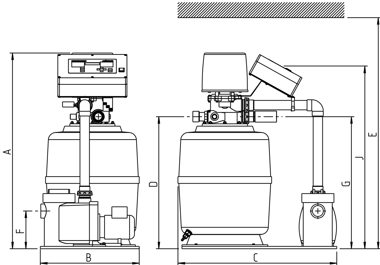
Abb. C-3: Maßzeichnung Filteranlage GENO-mat® F 500 A
