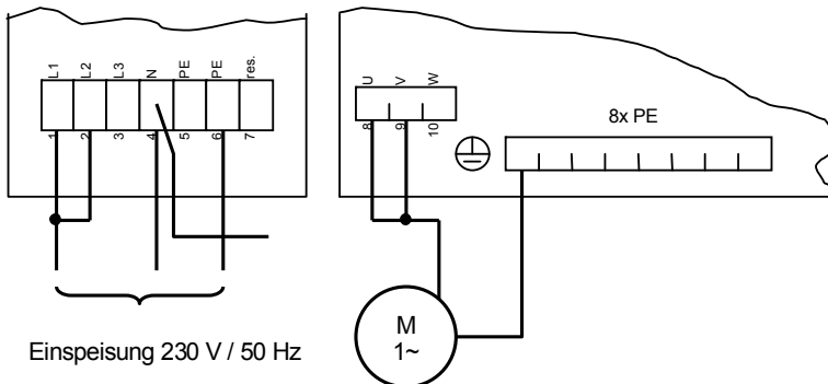
Abb. D-4: Anschlussbeispiele der Umwälzpumpe
