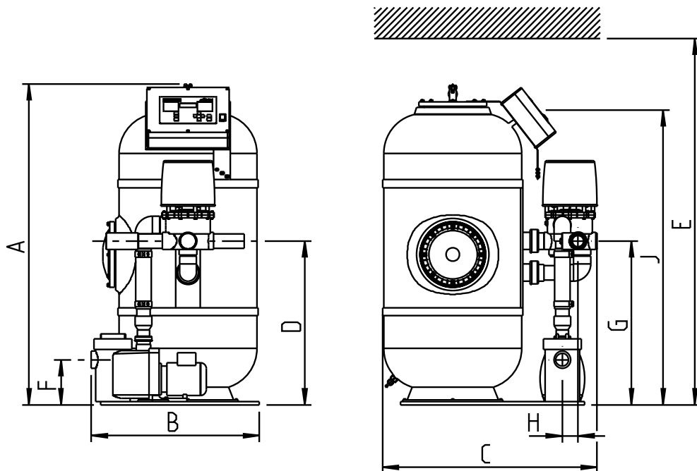
Abb. C-4: Aufstellung: Filteranlage GENO-mat® F 600/610 A
