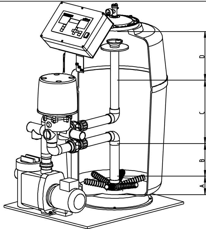
Abb. D-2: Schüttschema zum GENO-mat® F 600 A
