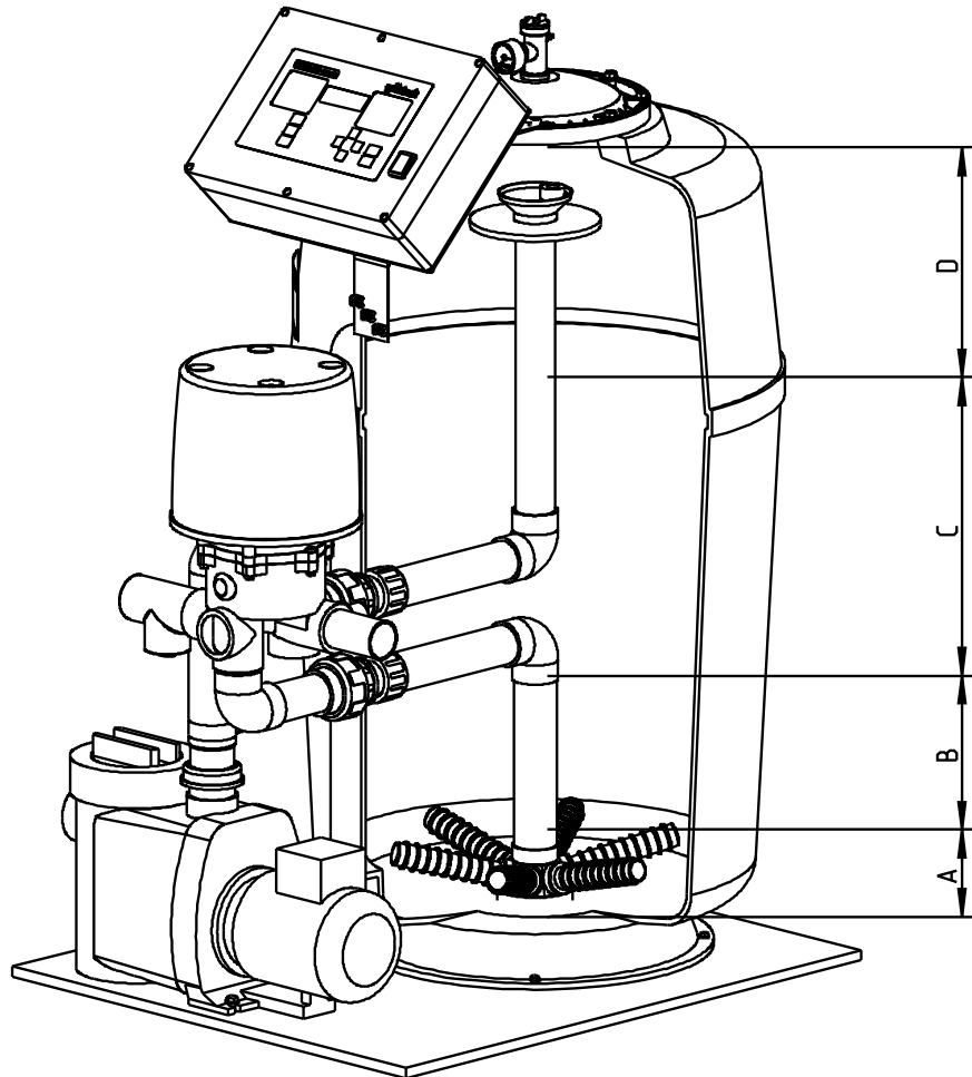
Abb. C-5: Schüttschema zu GENO-mat® F 600 A
